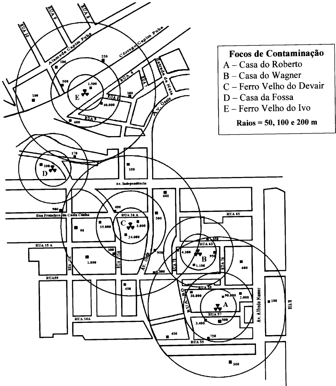
Figura 1. Avaliação da atividade de ^{137}\text{Cs} em Bq/kg nos solos superficiais do Bairro Setor Aeroporto - Goiânia, feita em dezembro de 1987 [2].
